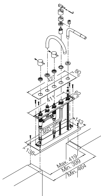
Uden monterageramme og box (BK-A system)
