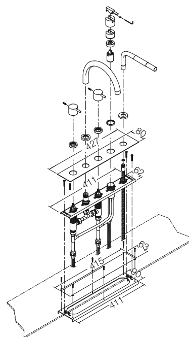
Til montage direkte på badekarkant (BK-B system)
